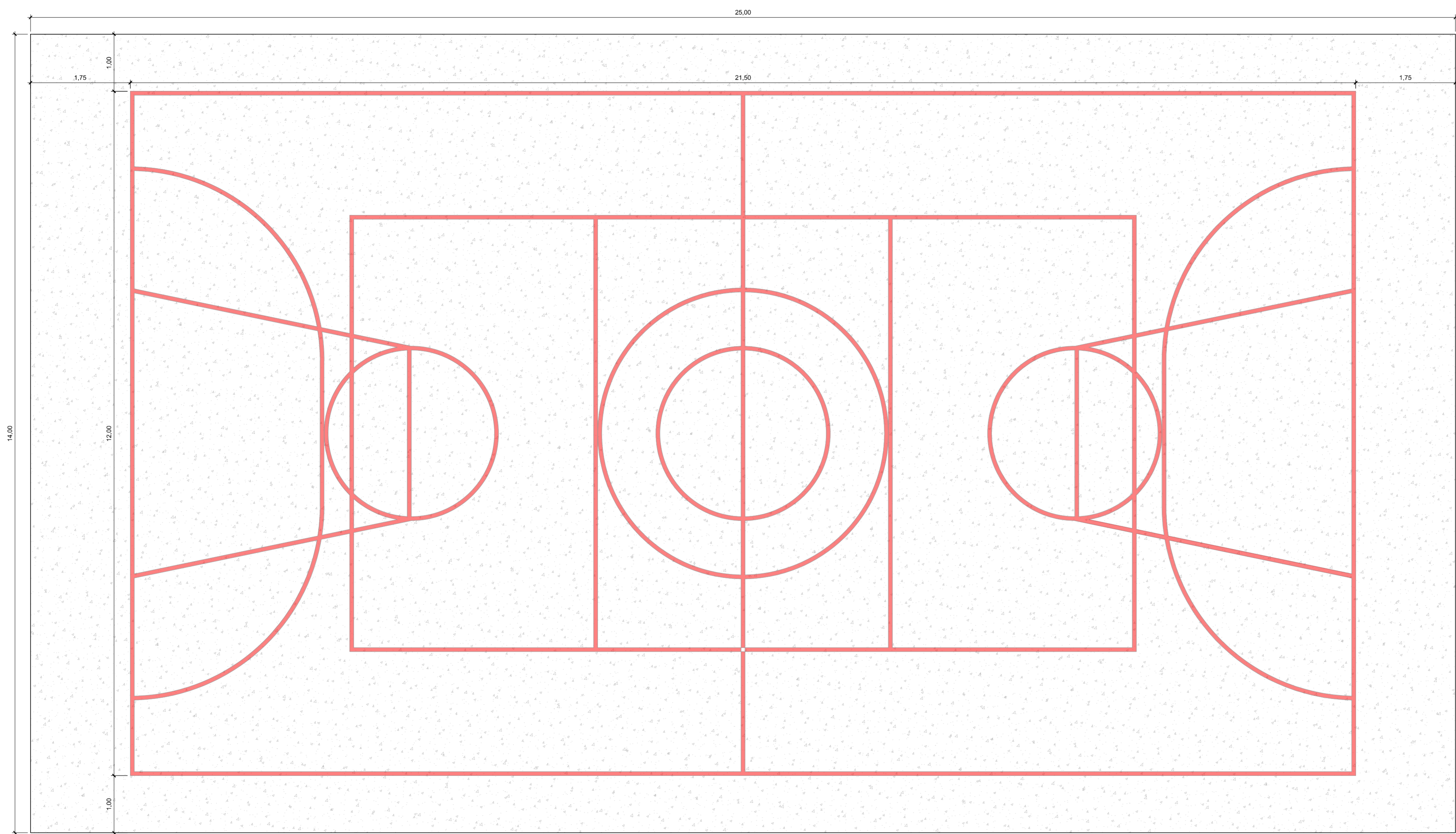
PLANTA BAIXA - MEDIDAS ESCALA 1:50
