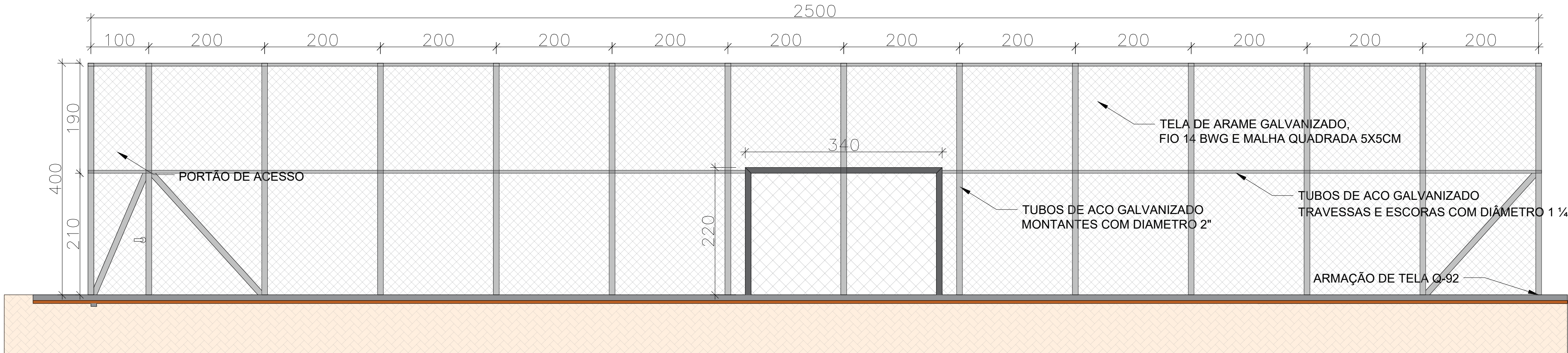
VISTA - GOLEIRA ESCALA 1:50
