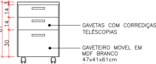
VISTA FRONTAL ESC. 1:20
