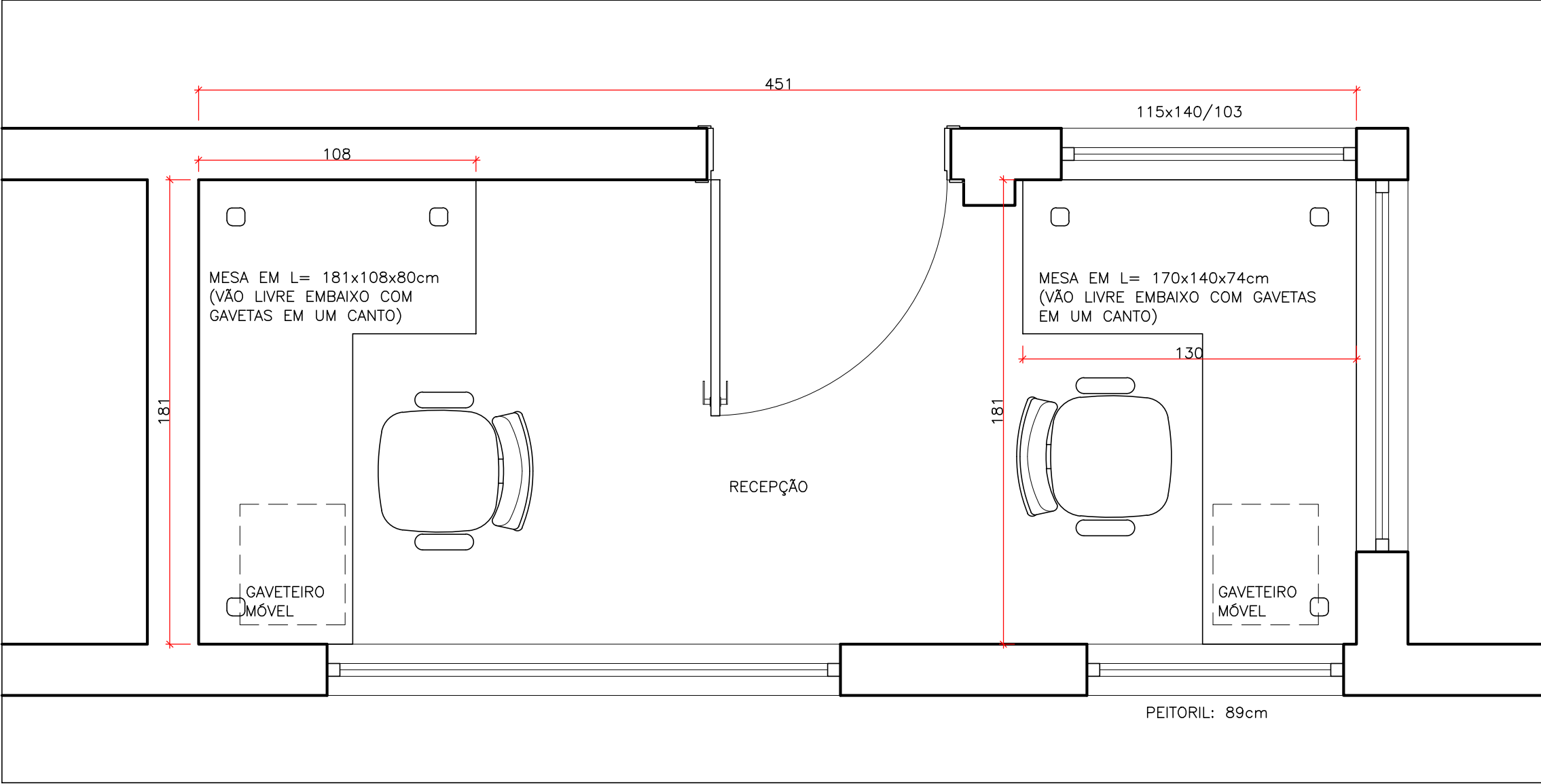
RECEPÇÃO – PLANTA BAIXA ESC. 1:20
