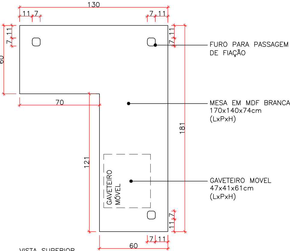
VISTA SUPERIOR ESC. 1:20
