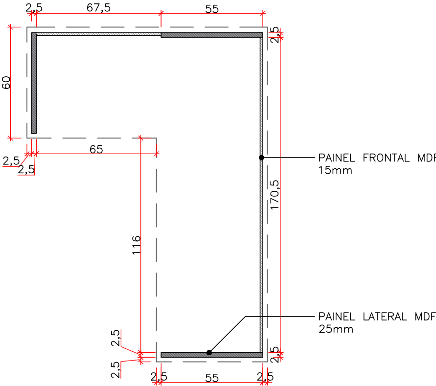
CORTE SUPERIOR ESC. 1:20
