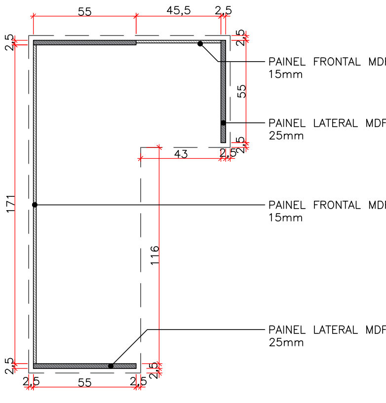
CORTE SUPERIOR ESC. 1:20
