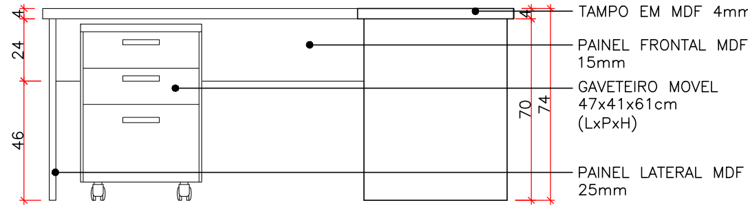
VISTA FRONTAL ESC. 1:20
