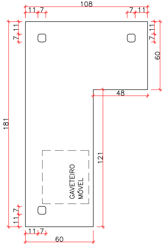
VISTA SUPERIOR ESC. 1:20
