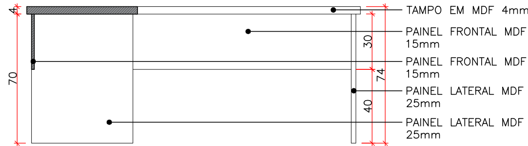
CORTE FRONTAL ESC. 1:20
