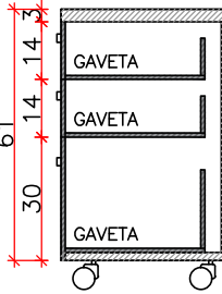
CORTE LATERAL ESC. 1:20
