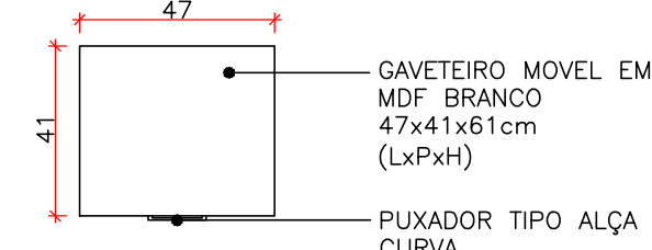
VISTA SUPERIOR ESC. 1:20
