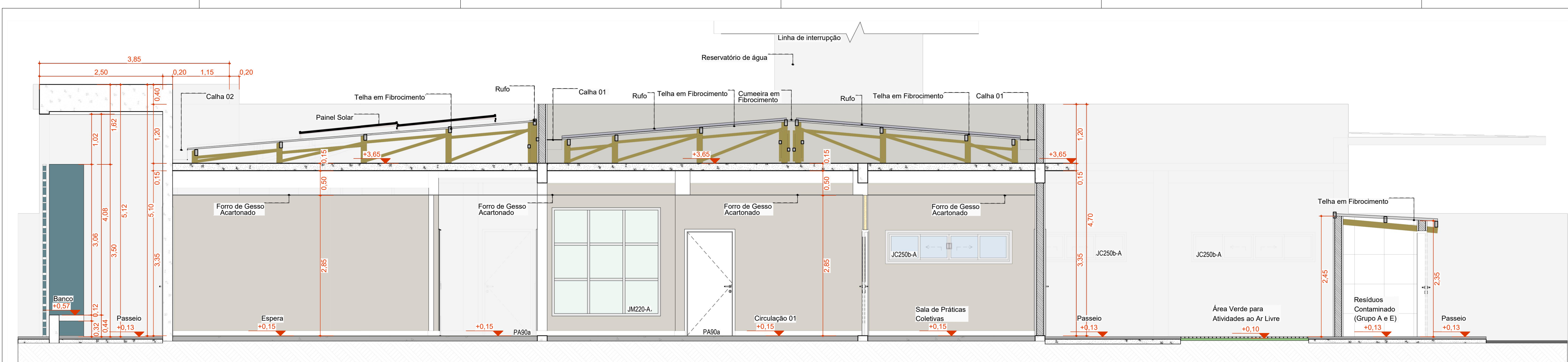
A Corte AA Escala: 1:50
