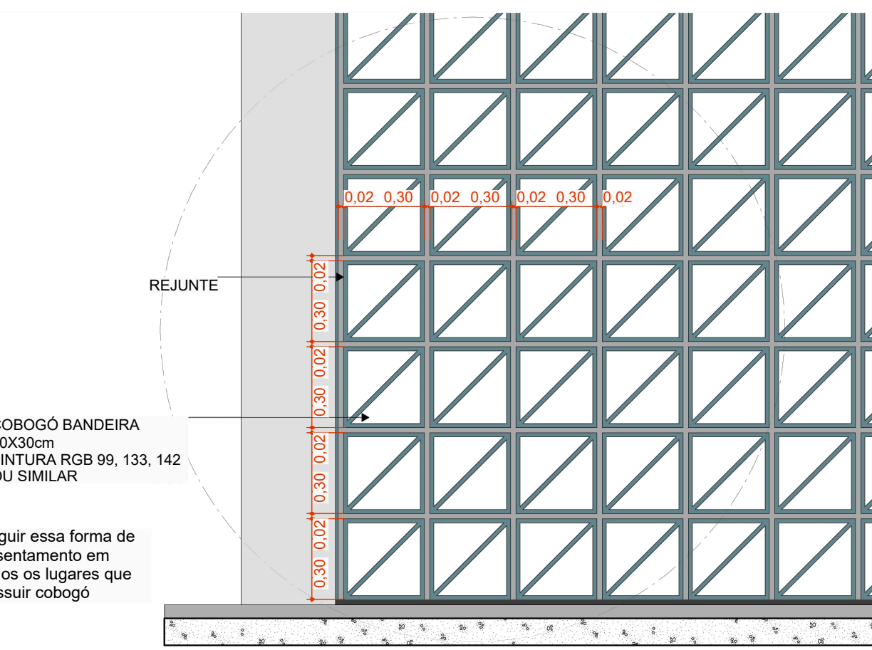
Detalhamento do assentamento do Cobogó Escala: 1:20
