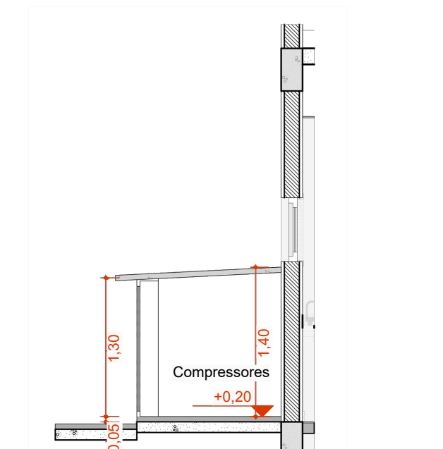
E Corte EE Escala: 1:50
