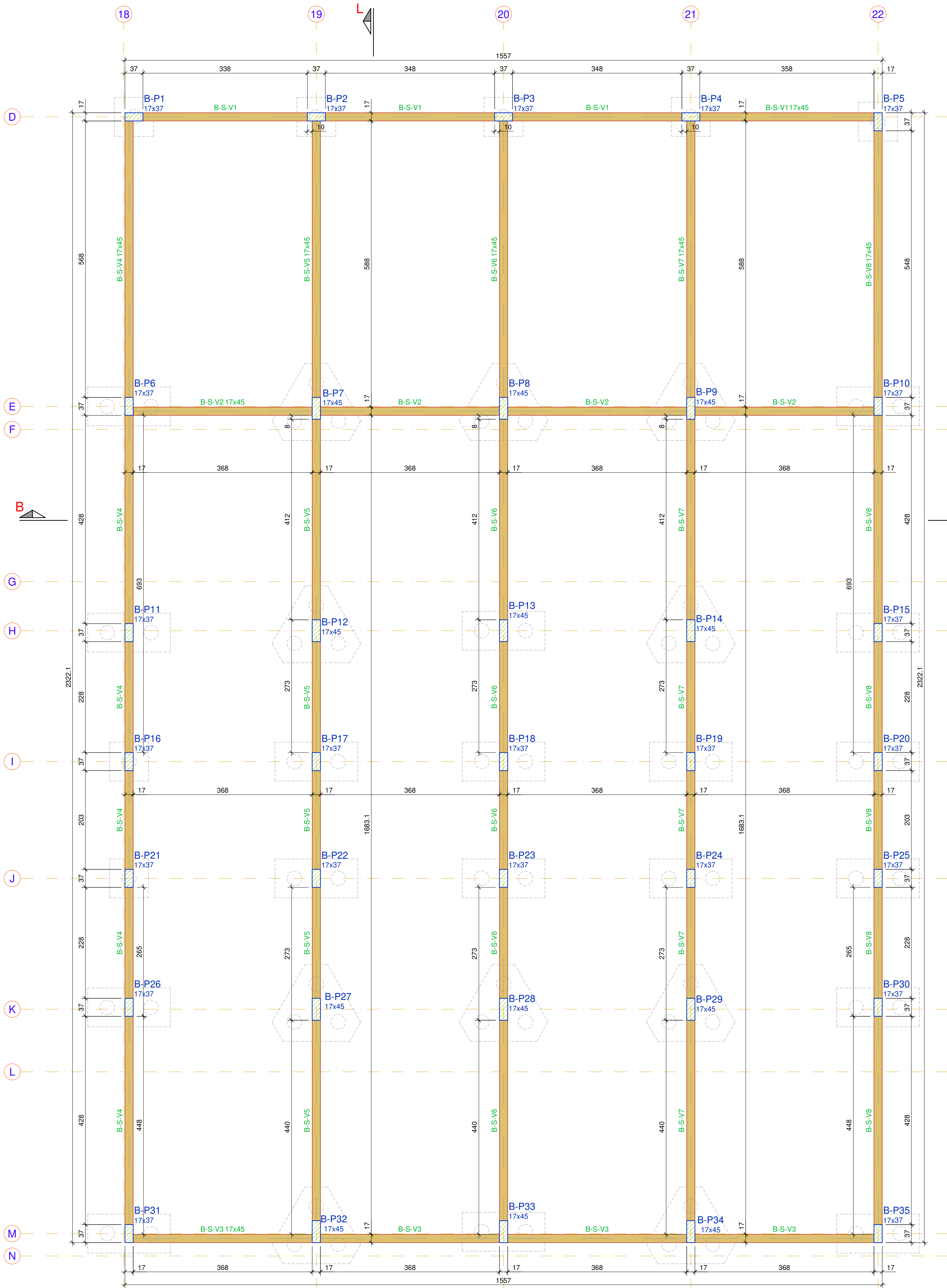
BLOCO B - FORMA - SUBSOLO ESCALA: 1/50
