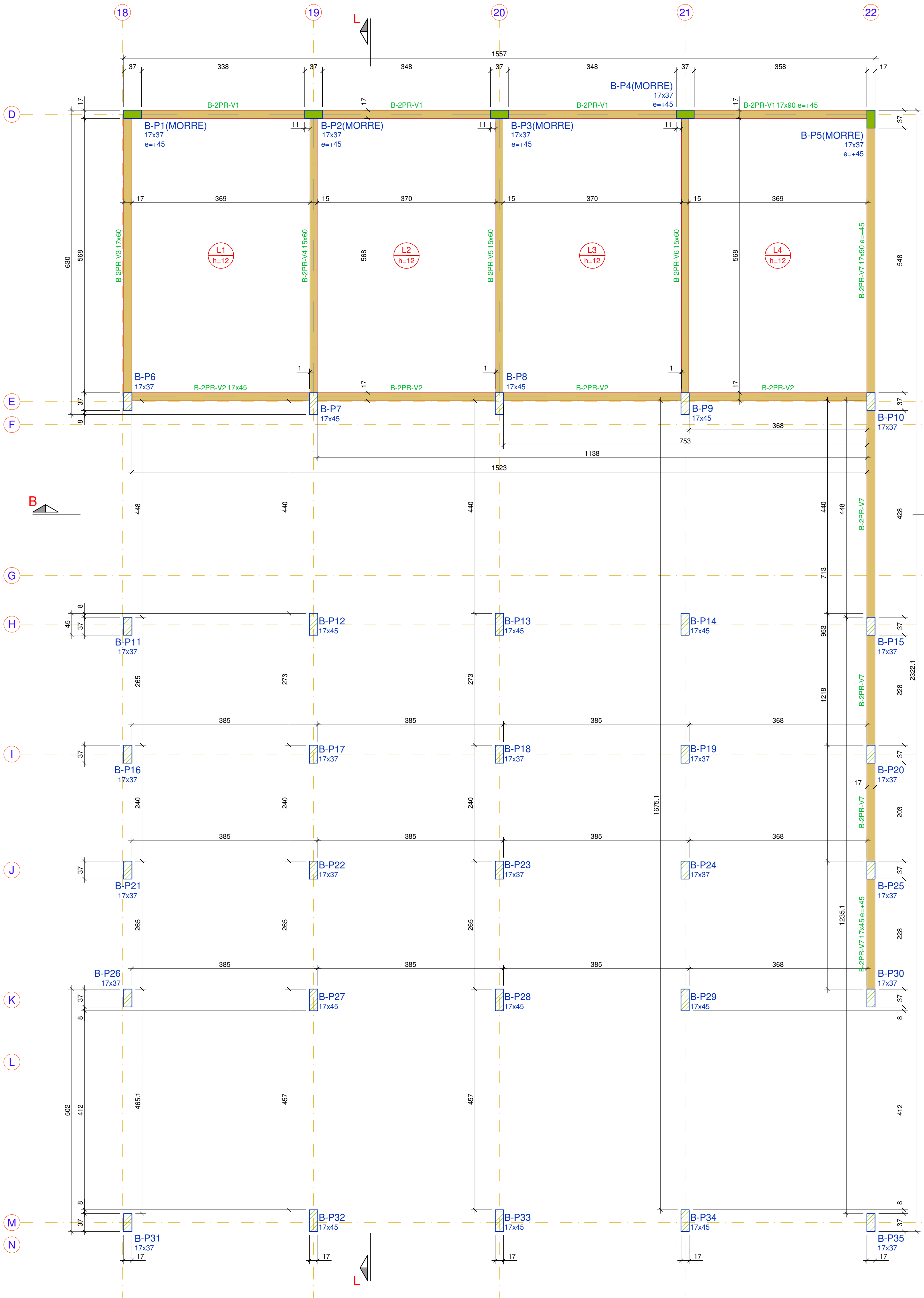
BLOCO B - FORMA - 2º PAVIMENTO REBAIXADO ESCALA: 1/50
