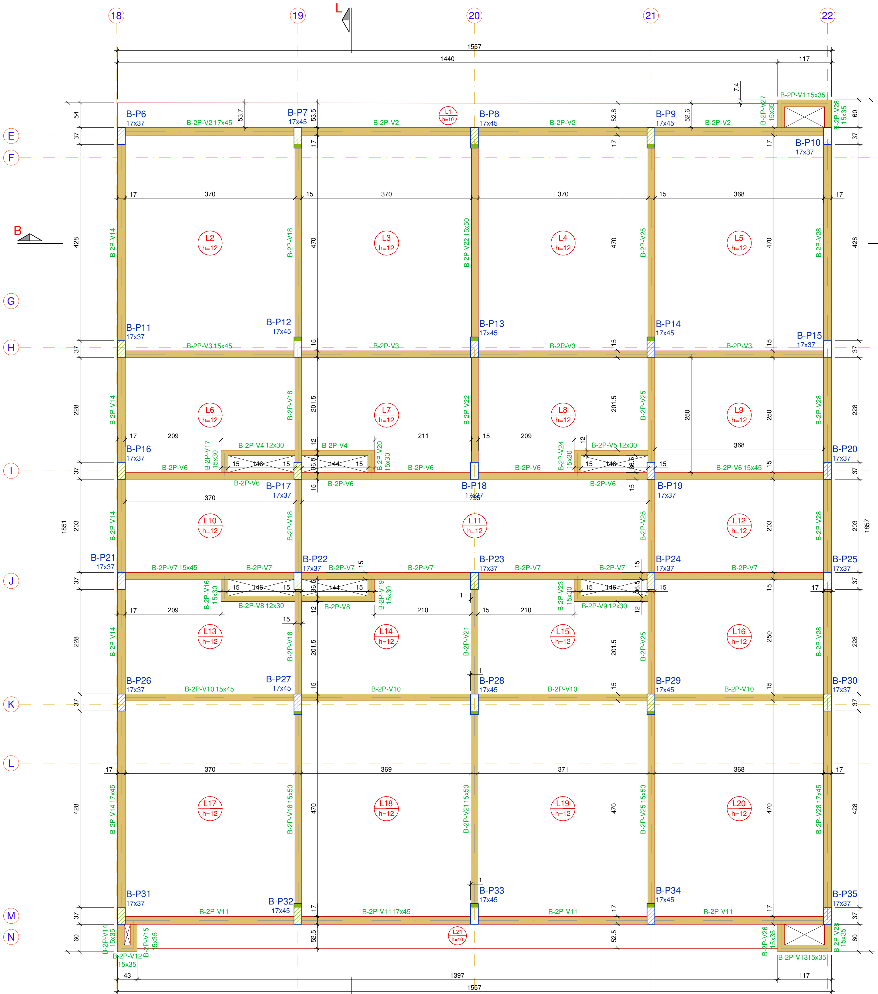
BLOCO B - FORMA - 2º PAVIMENTO ESCALA: 1/50
