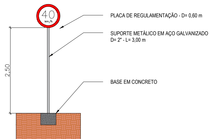
5 Detalhamento Placas de Sinalização ESC: s/escala
