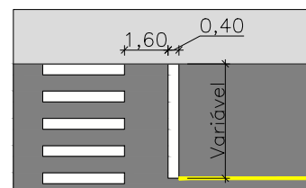
6 Detalhamento Linha de Retenção ESC: s/escala
