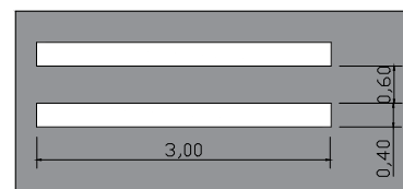
3 Detalhamento Faixa de Pedestre ESC: s/escala
