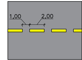
7 Detalhamento Pintura - Faixa Seccionada ESC: s/escala
