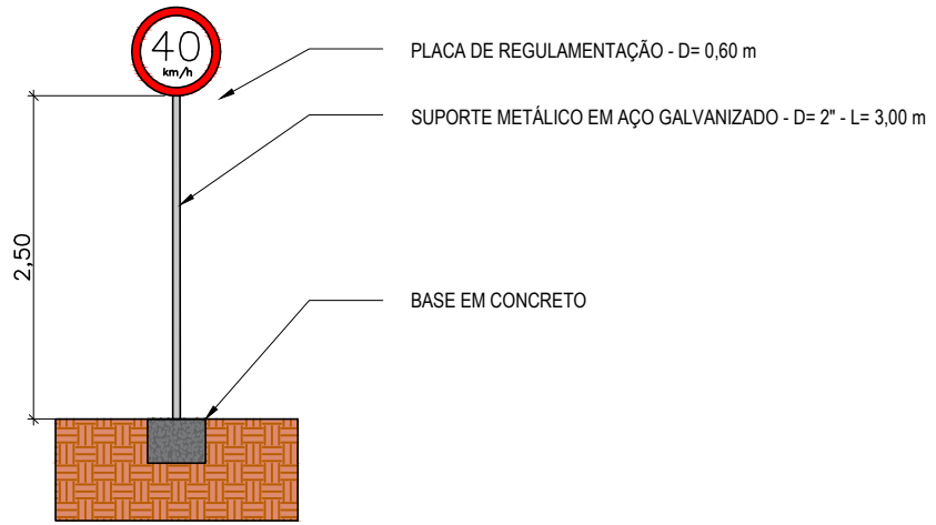
5 Detalhamento Placas de Sinalização ESC: s/escala
