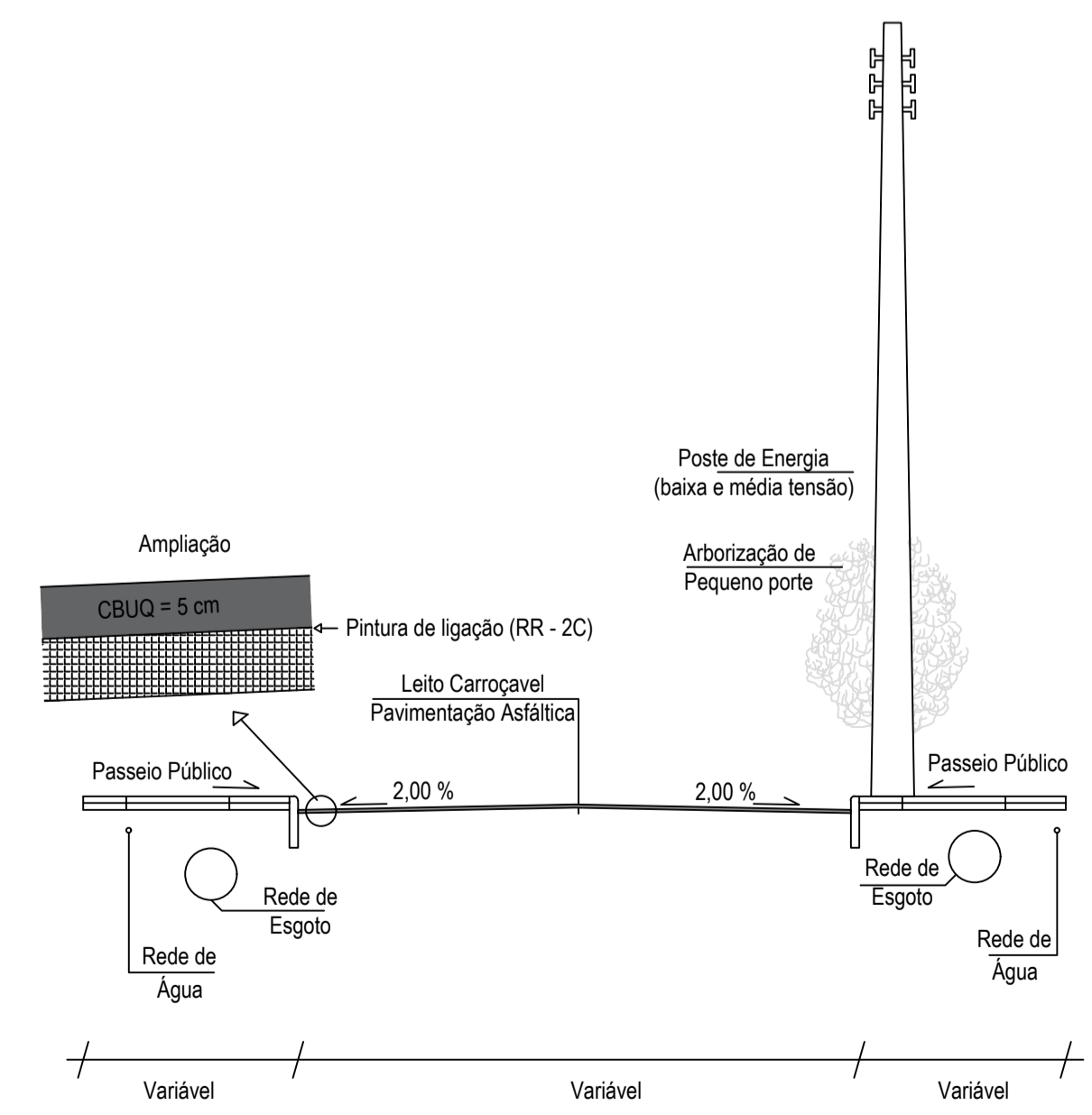
3 Corte Esquemático ESC: s/escala
